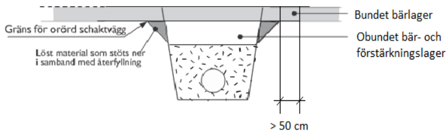
Figur 2. Tvärsektion på återställning
